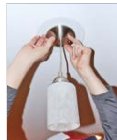
WIRE & INSTALL PENDANT CANOPY
